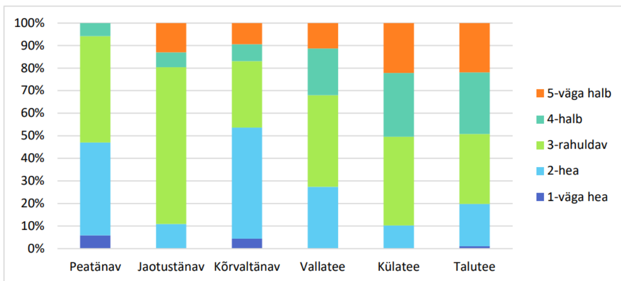
Joonis 19: Teekatte seisukord teedel ja tänavatel (allikas: Häädemeeste valla teehoiukava 2025-2029)
