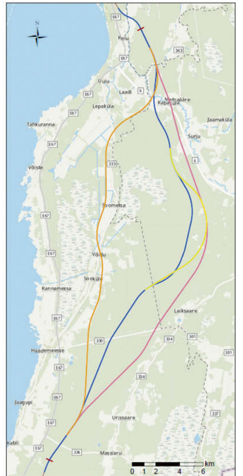
Joonis 1. Rail Balticu kuus trassialternatiivi, mida omavahel võrreldi ja hinnati
